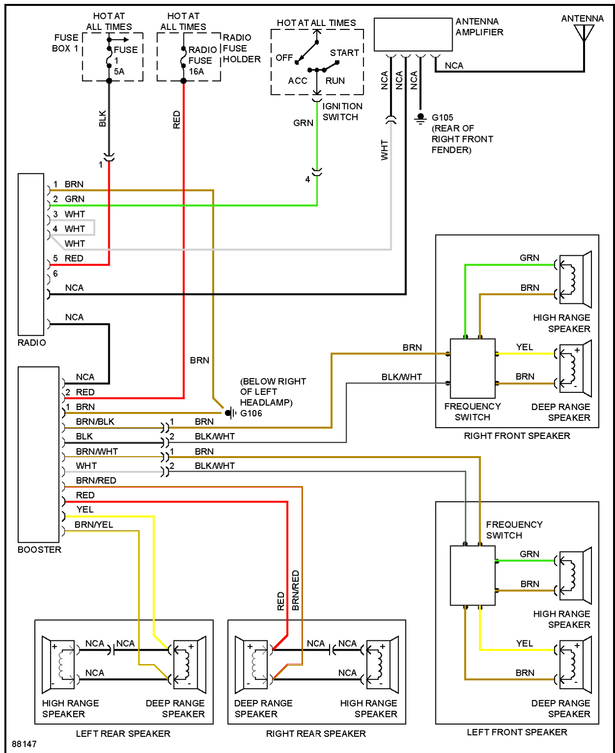
Fig. 9: Radio Circuits
